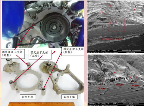
圖二 鼓風機齒盤相固 定座支架斷裂件拆檢前 SEM斷面（上）及放大的外觀（圖）
